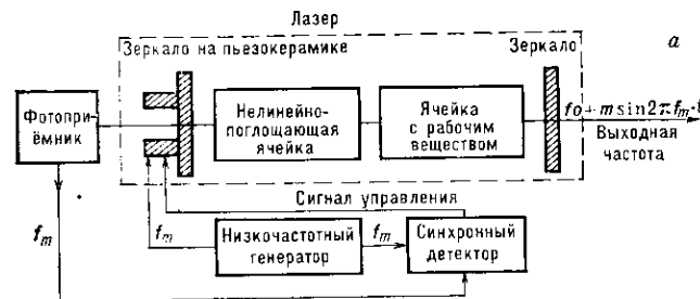
Рис. 3. Блок-схема оптического стандарта частоты: а — внешний репер; б — внутренний. Автоподстроика резонатора необходима для уменьшения эффекта затягивания частоты.
