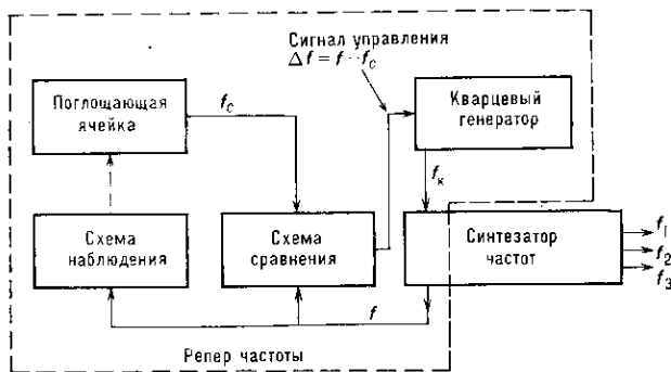
Рис. 2. Блок-схема пассивного стандарта частот.
